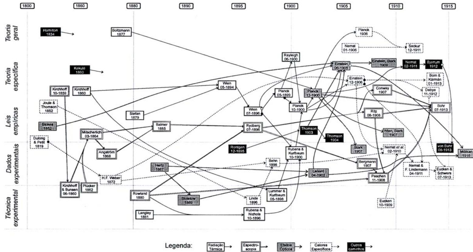
FIGURA 7: Rede de influências entre artigos levando aos primórdios da Física Quântica Velha.
